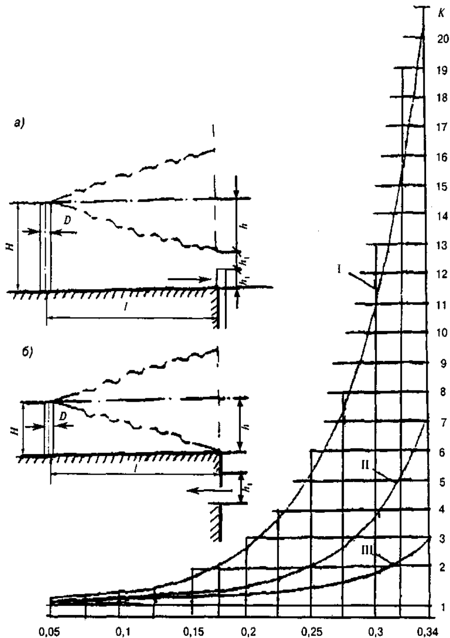
а - расположение источника над зоной всасывания наружного воздуха приемным устройством (высота трубы источника H = 2h_1 + h ); б - то же, над кровлей здания (высота трубы источника H = h ); h - расстояние по вертикали, м, горизонтальной оси струи; h_1 - высота отверстия для приема наружного воздуха, м; l - расстояние между устьем источника и приемным устройством для наружного воздуха, м.
